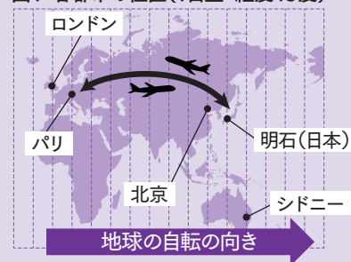
図1 各都市の位置(1目盛 経度15度)
